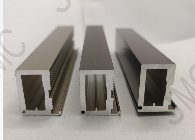
T6063 太阳能边框 Solar Border
